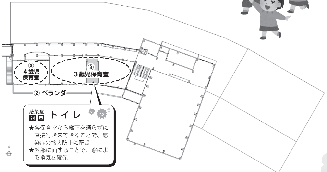
ひまわり保育園増築棟（平面図）
